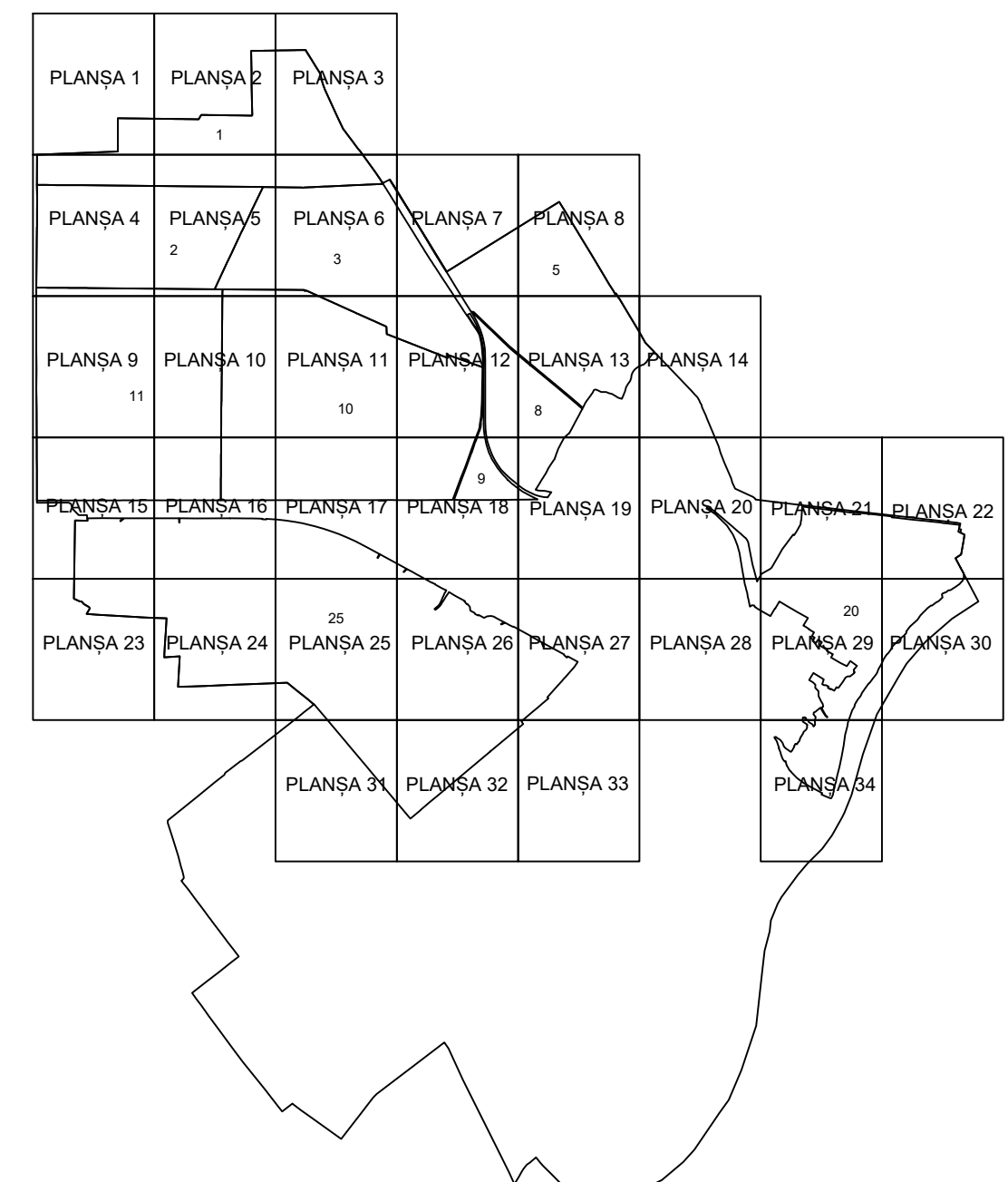
Schema planșelor
