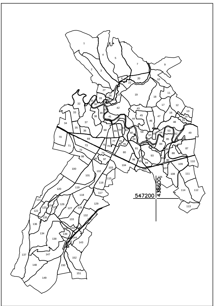
SCHITA CU DISPUNEREA SECTOARELOR CADASTRALE
