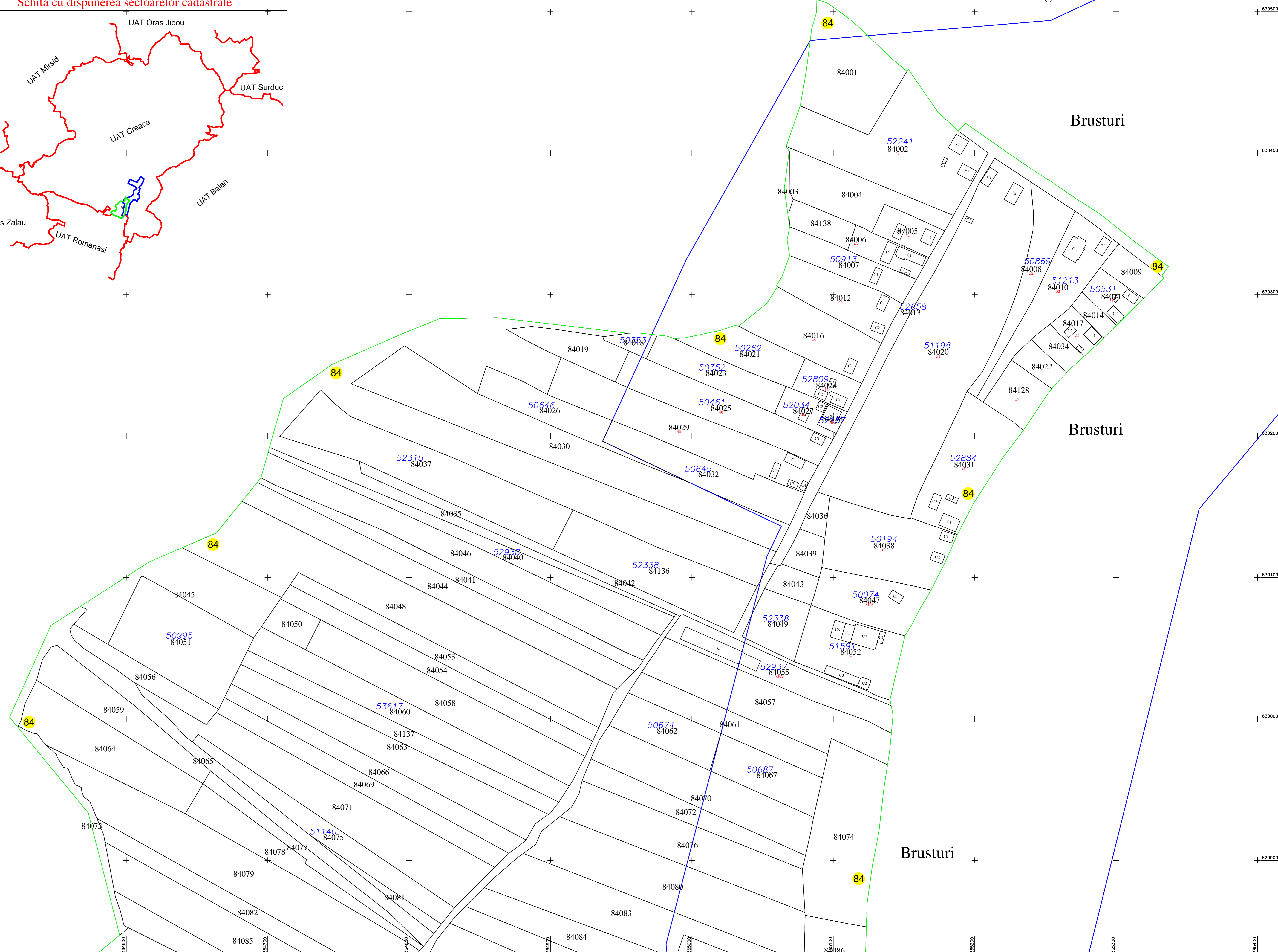
Schita cu dispunerea sectoarelor cadastrale
