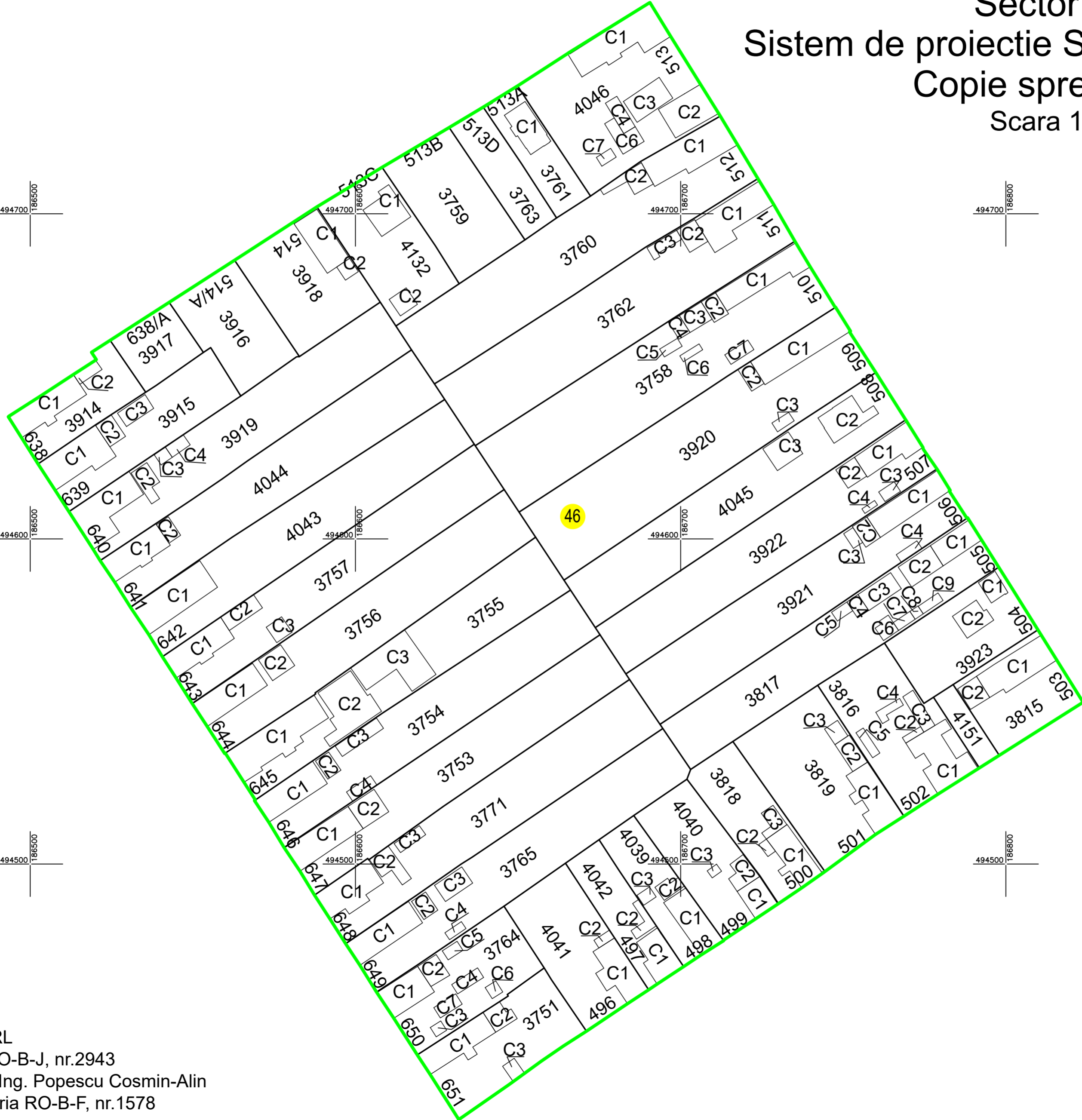
Schița de dispunere a sectoarelor cadastrale UAT Biled
