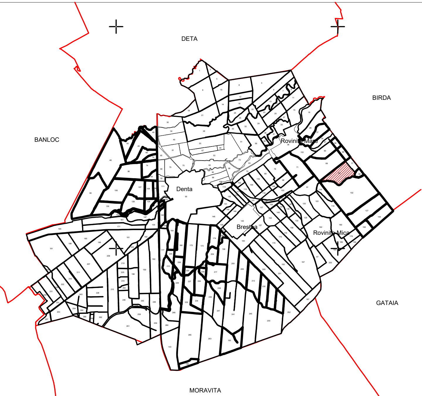
Schita de dispunere a sectoarelor cadastrale UAT DENTA
