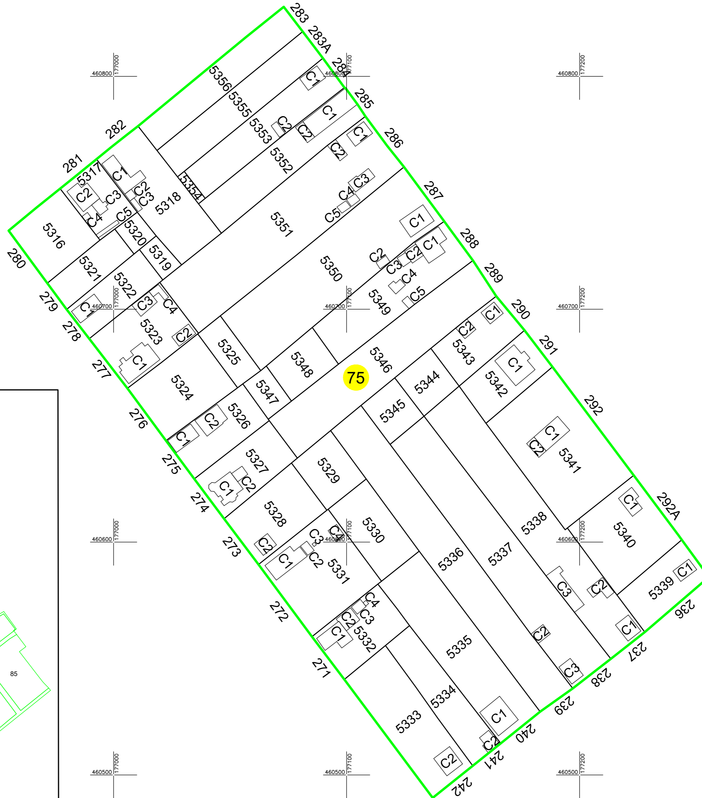
Schita de dispunere a sectoarelor cadastrale Localitatea Iohanisfeld, Comuna Otelec
